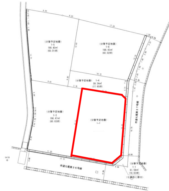
測量図
